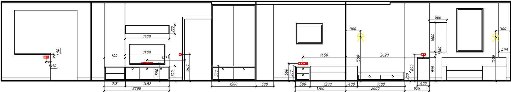
Развертка стен лоджии
