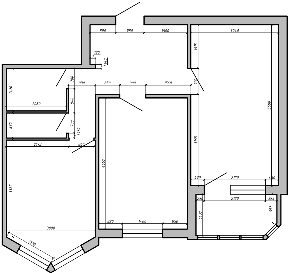
Обмерный план
