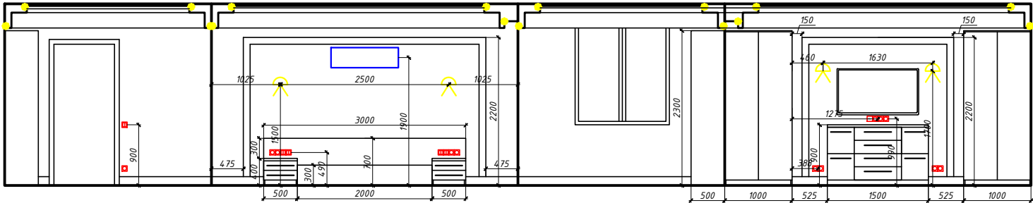
Развертка стен спальни
