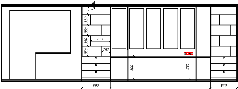
Развертка стен спальни
